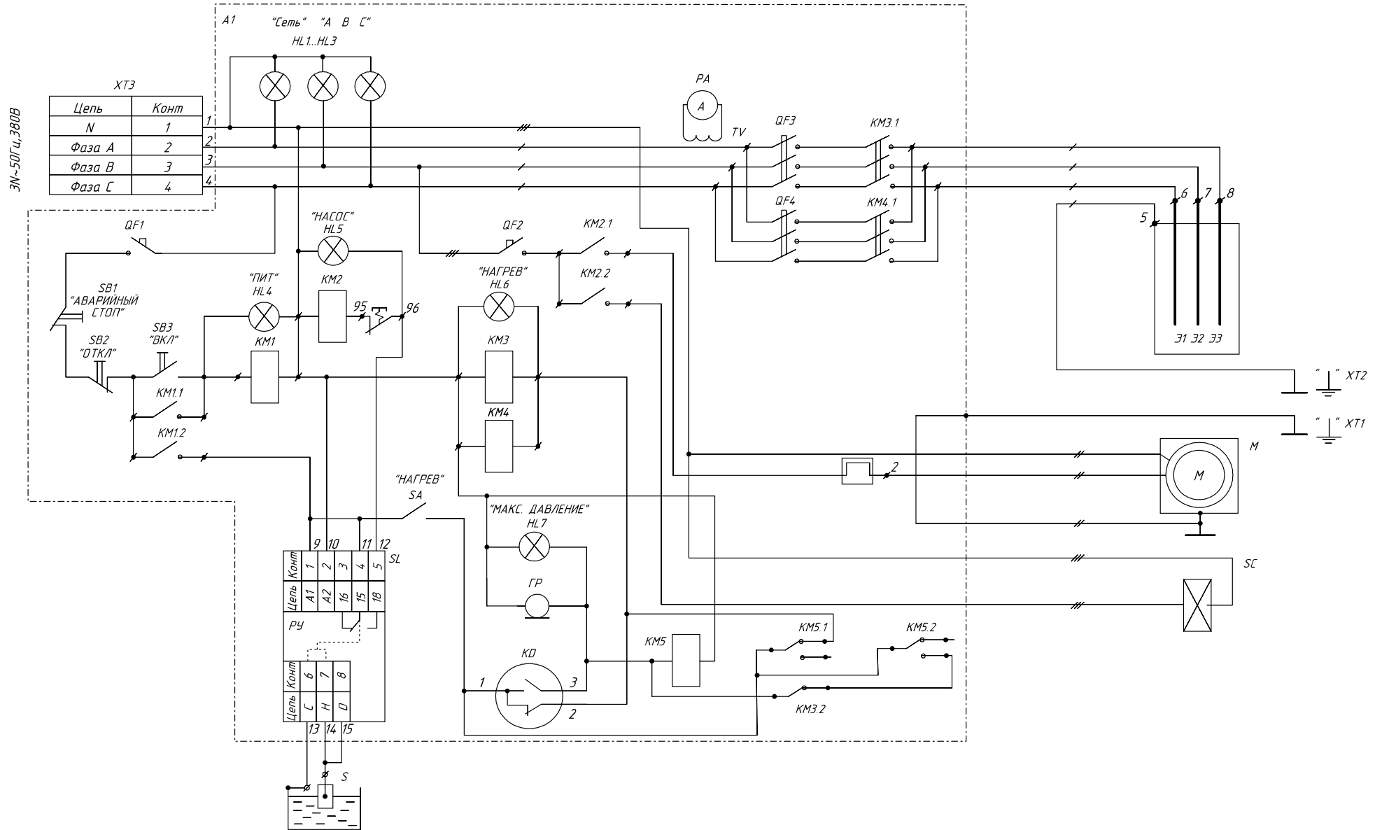
Рисунок 3 - Парогенератор ИПКС-129-50, ИПКС-129-100. ИПКС 129.03.00.000-01Э3 Схема электрическая принципиальная.
