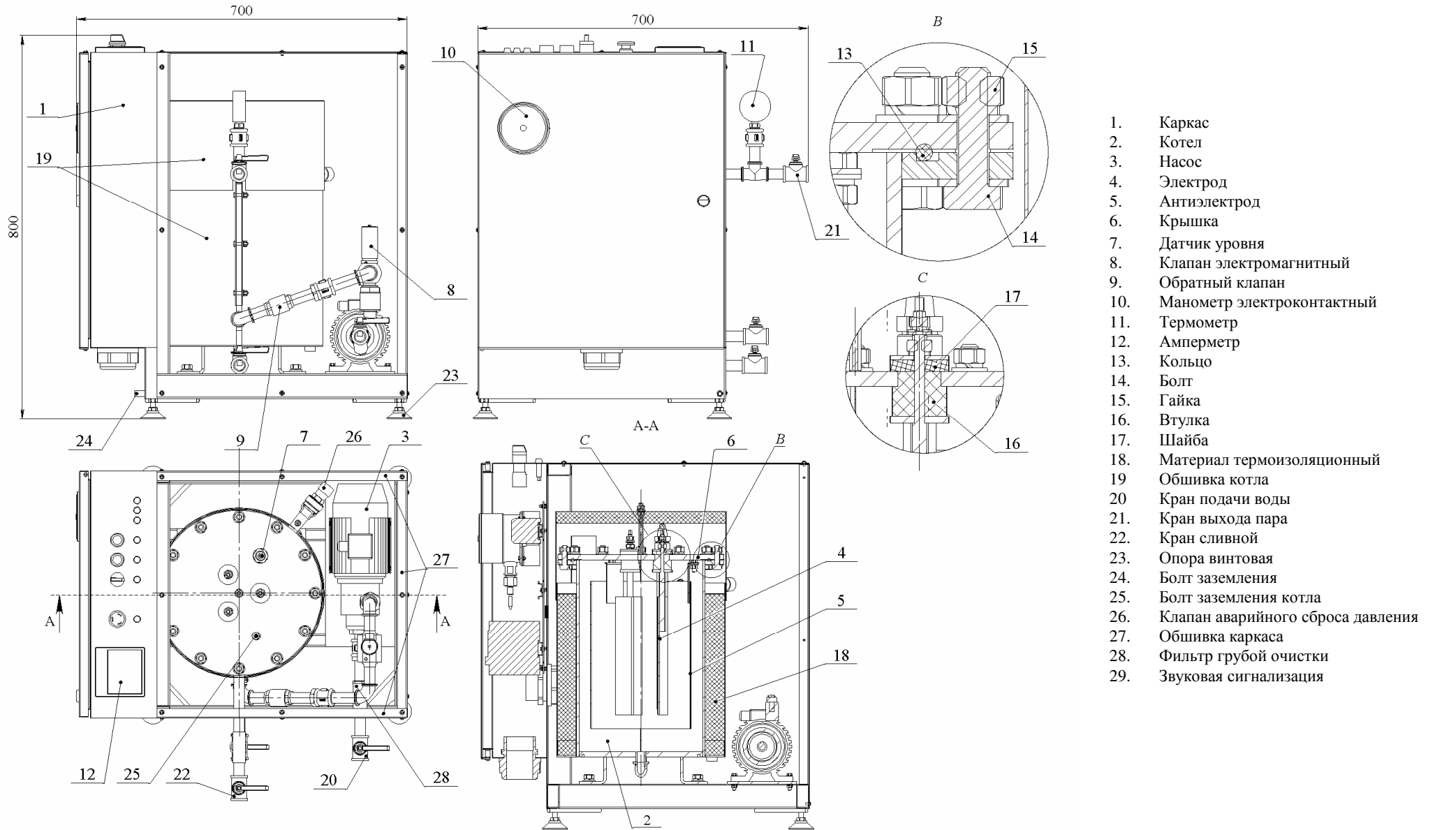
Рисунок 1 – Парогенератор ИПКС-129-50, ИПКС-129-100.
